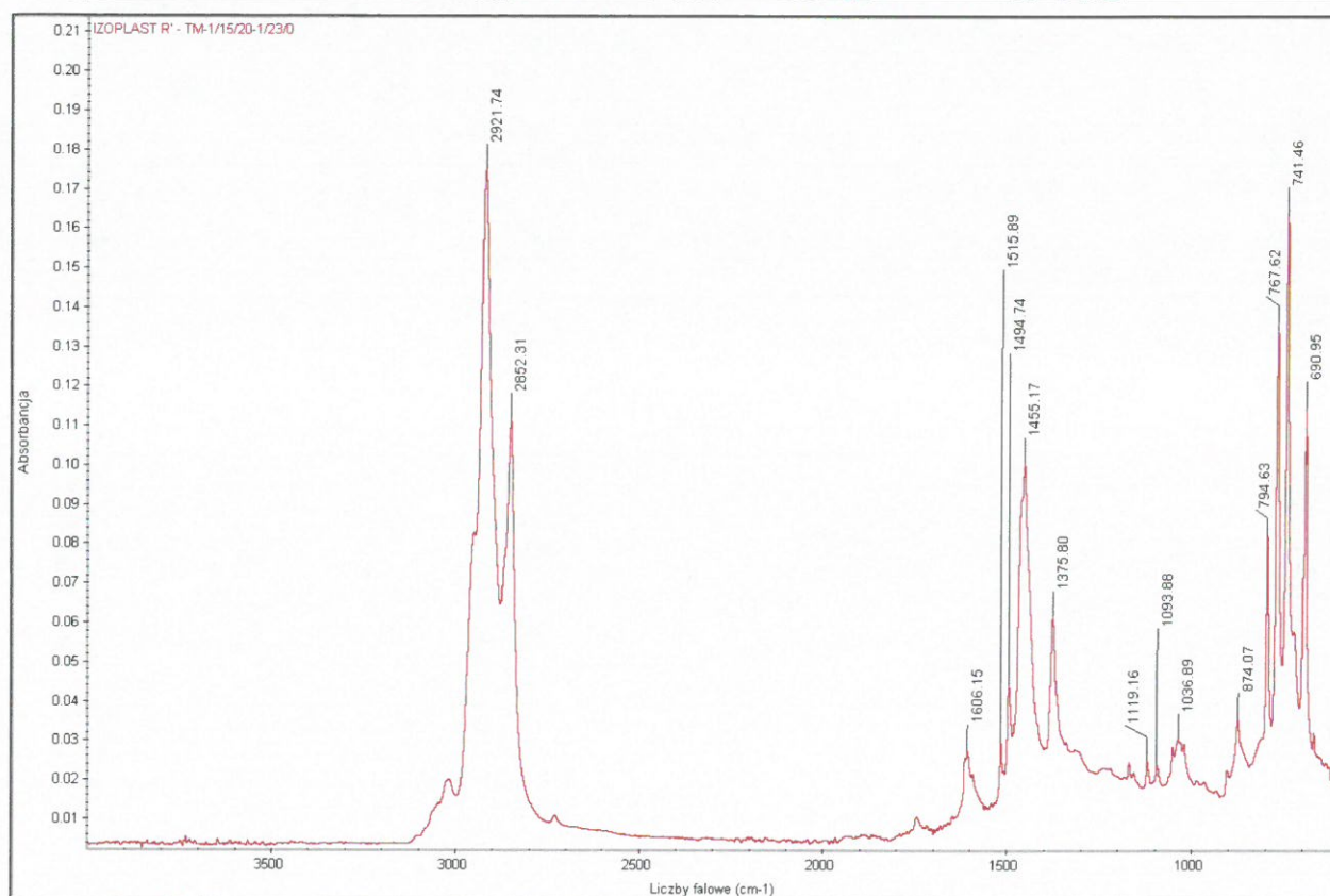
Rysunek 1– Widmo w podczerwieni (analiza FTIR) roztworu asfaltowego IZOPLAST R'
